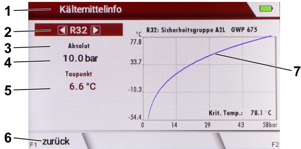
Bild Kältemittelinfo
