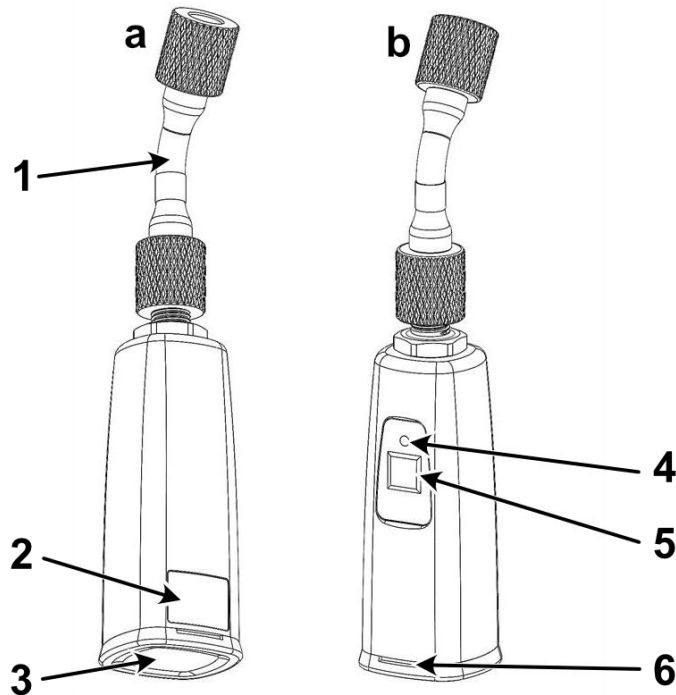
Kabelloser Drucksensor
